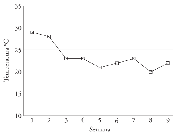
Figura 2. Evolución de la temperatura en los vermireactores. Figure 2. Temperature changes in vermireactors.
