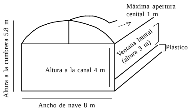
Figura 1. Dimensiones de la estructura de un módulo del invernadero con apertura cenital ala de gaviota.
