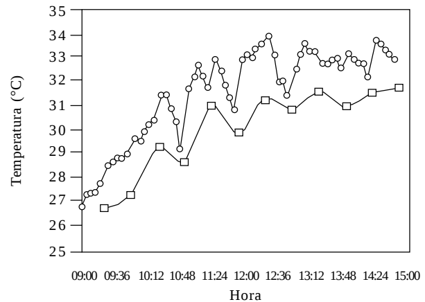
Figura 2. Dinámica de temperatura dentro (○) y fuera (□) del invernadero en un día soleado.
